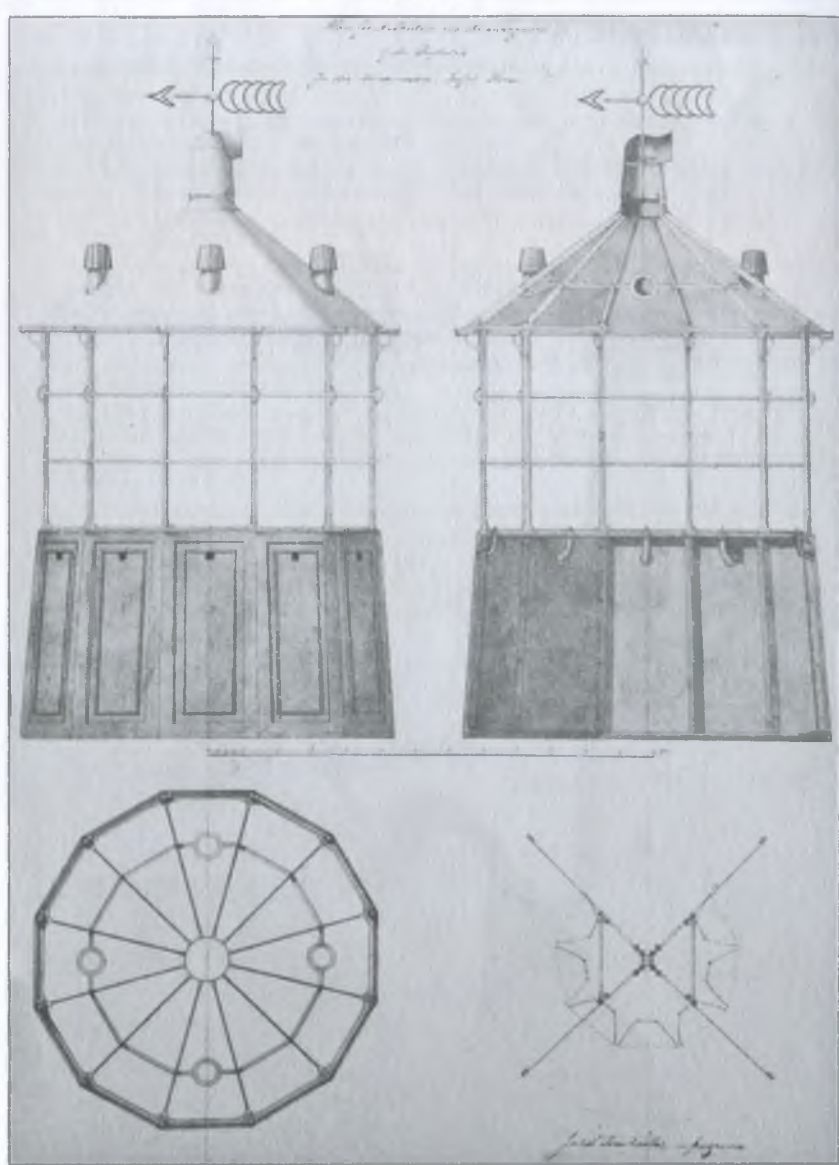
Копия чертежа Нижне-Бердянского маяка на Дальней косе.
